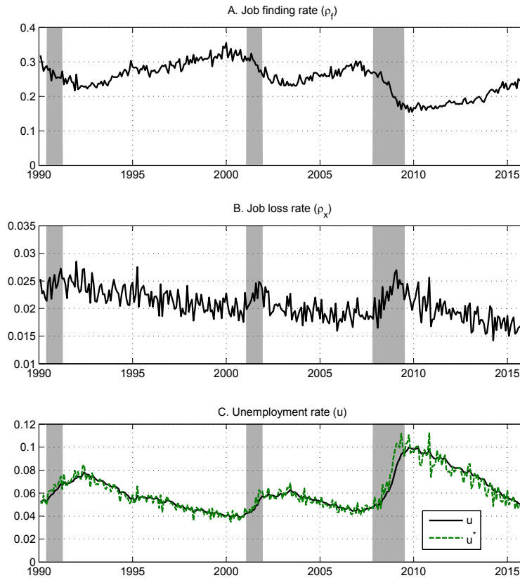
Figure 2: Raw data.
